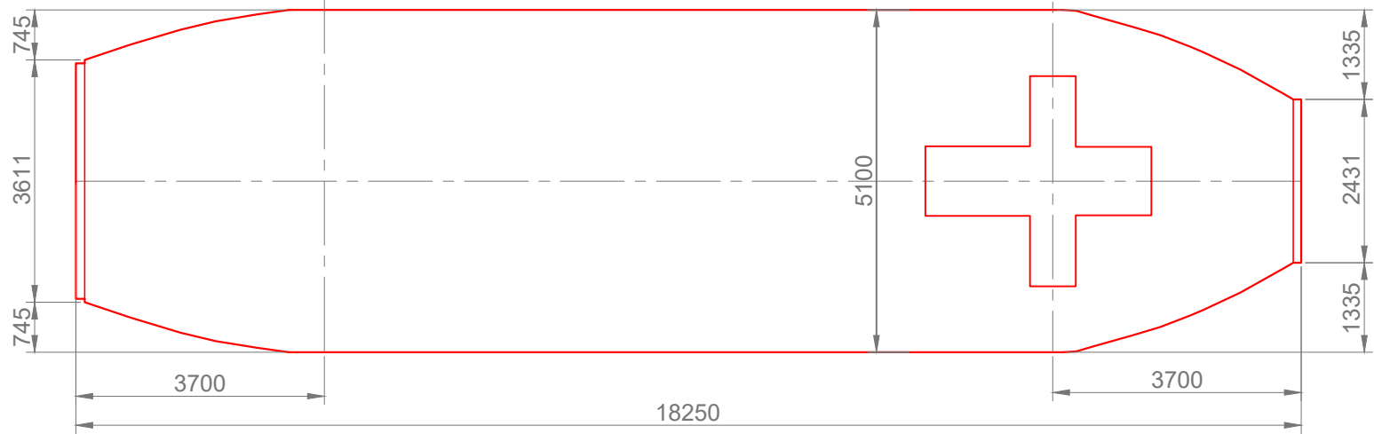
Bovenaanzicht Schaal 1:100
